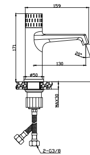
MONOCOMANDO LAV.
