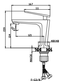
MONOCOMANDO LAV.
