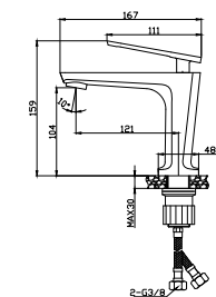
MONOCOMANDO BIDÉ
