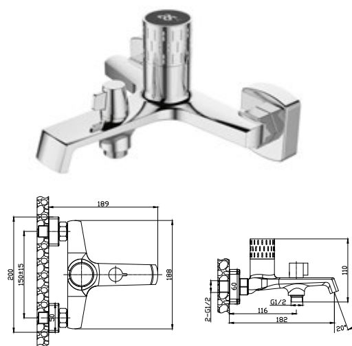
MONOCOMANDO BANHEIRA
