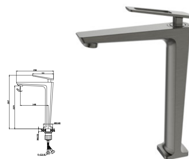
MONOCOMANDO LAV.
