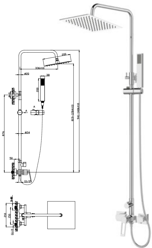
RAMPA CHUVEIRO
