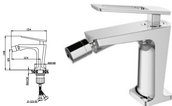
MONOCOMANDO BIDÉ
