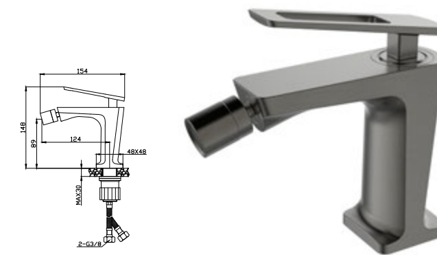
MONOCOMANDO LAV.
