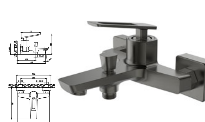
MONOCOMANDO BANHEIRA
