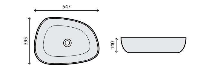
RS78547 Dim.: 54,7 x 39,5 x 14 cm Pack: 11 kg / 0,038 m³
