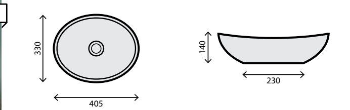
RS7138MW Dim.: 40,5 x 33 x 14 cm Pack: 6kg / 0,03m³
