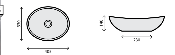
RS7138 Dim.: 40,5 x 33 x 14 cm Pack: 6kg / 0,03m³
