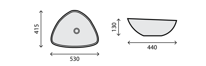
RS78015 Dim.: 53 x 41,5 x 13 cm Pack: 9,5kg / 0,035m³
