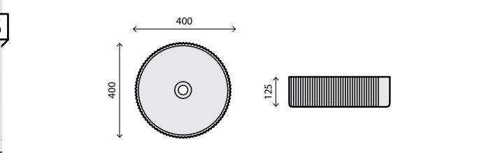
RS545 - Totalmente Gloss Dim.: Ø 40 x 12,5 cm Pack: 10 kg / 0,025 m³
