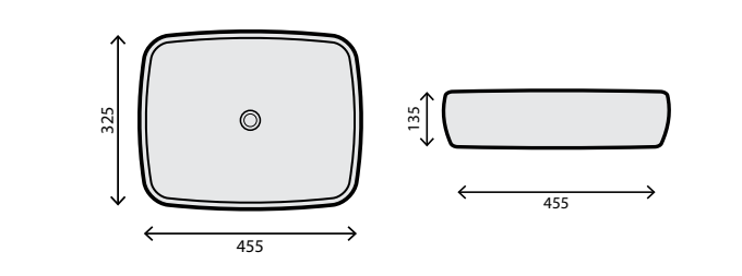
RS78105MCP Dim.: 45,5 x 32,5 x 13,5 cm Pack: 7 kg / 0,025 m³
