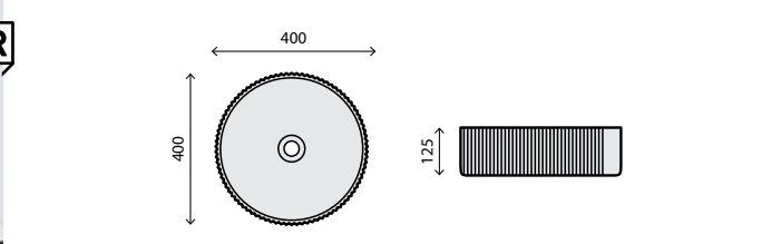
RS545ASBR - Asper + Mate Dim.: Ø 40 x 12,5 cm Pack: 10 kg / 0,025 m³
