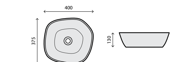
RS78563 Dim.: 40 x 37,5 x 13 cm Pack: 9kg / 0,036m³
